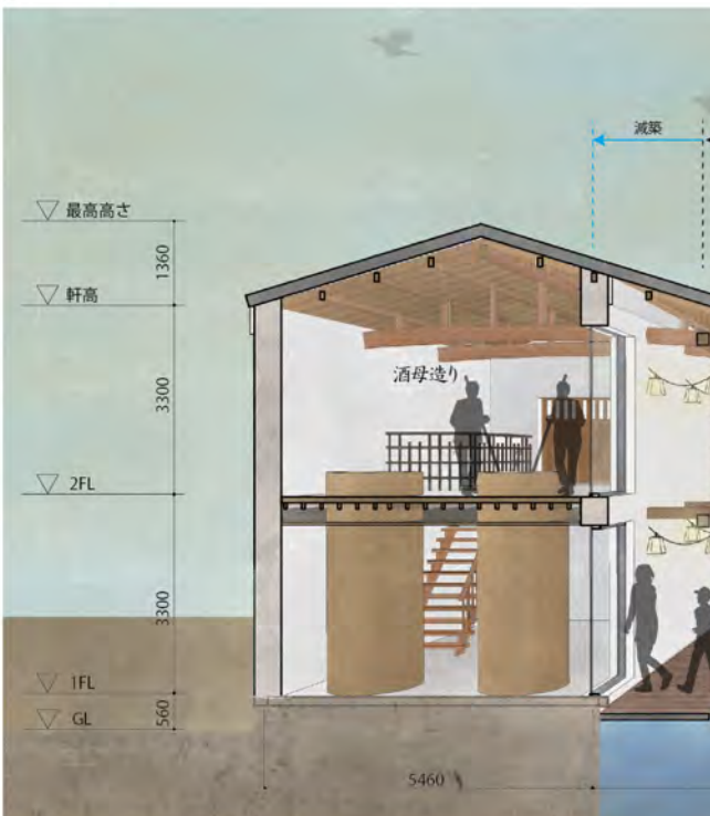
A断面図
